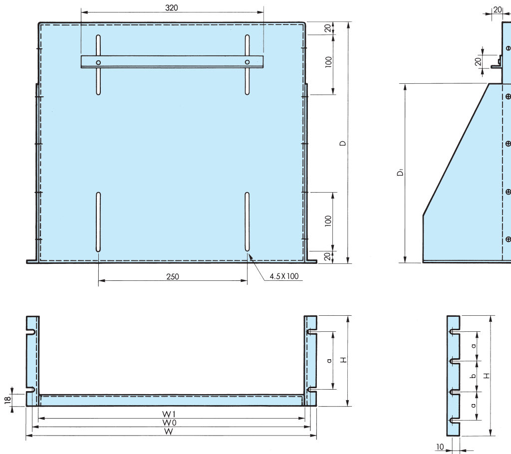
寸法図
