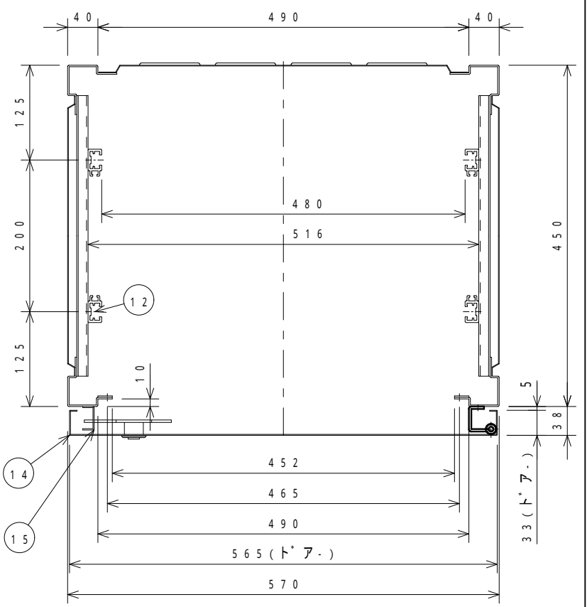
断面図 (1/5)
